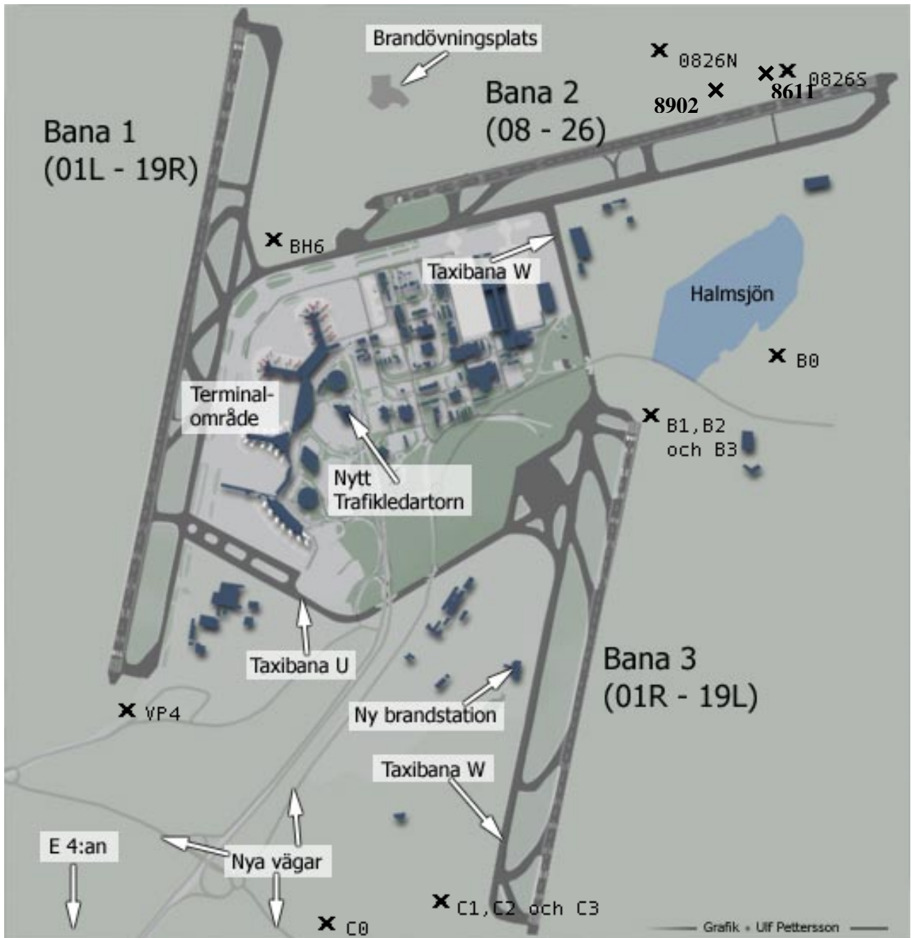
Figur 1: Lokalisering av kontrollbrunnar för grundvattenskydd vid Stockholm- Arlanda flygplats.
